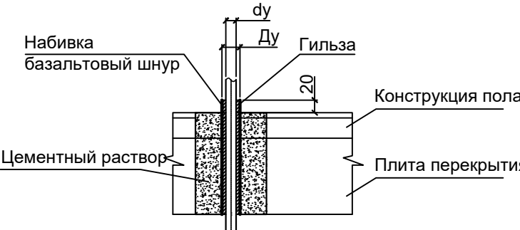
Узел прохода трубопровода через перекрытие
