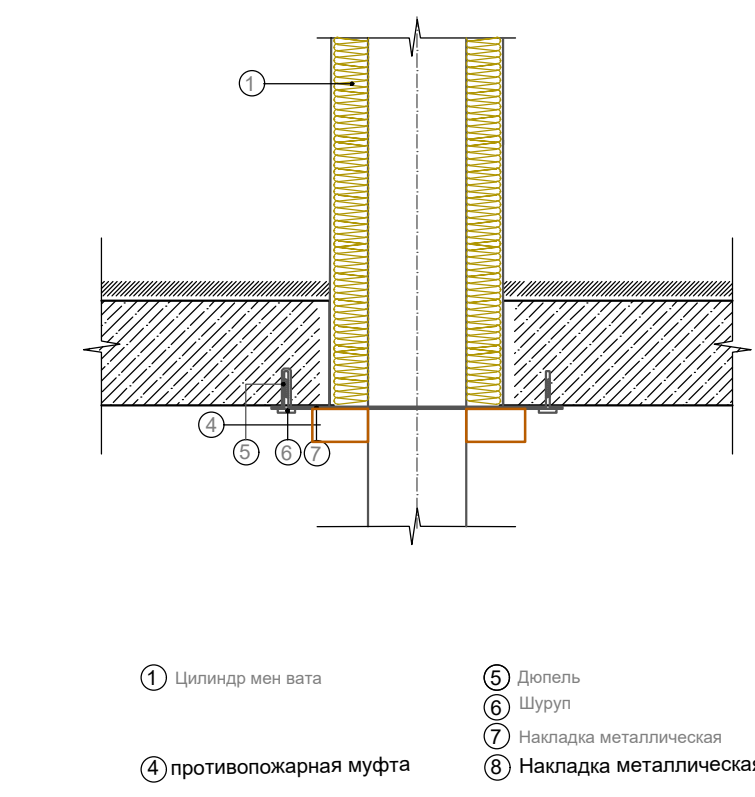
Типовой узел прохода трубопровода через перекрытие
